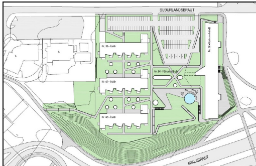
Hjúkrunarheimili í Sogamýri, afstöðumynd.
