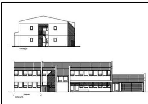
Sýsluskrifstofur Eskifirði, útlitsteikning.
