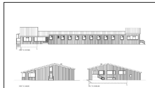
Fangelsi Kvíabryggju, útlit.
