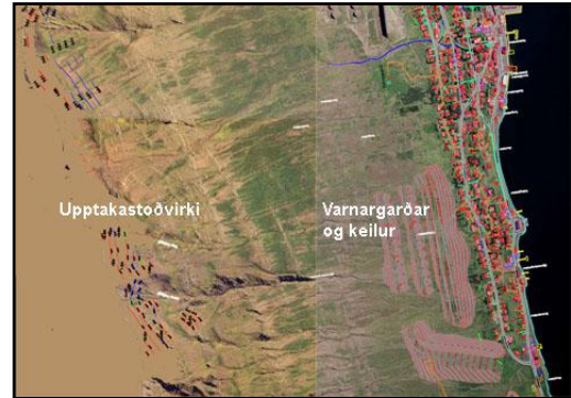
Yfirlit snjóflóðavarna í Tröllagili, Neskaupstað..
