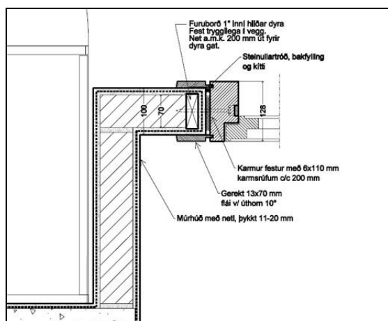
Deili af yfirfeldri hurð fangaklefa.
