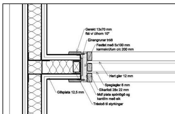
Deili af inniglugga.
