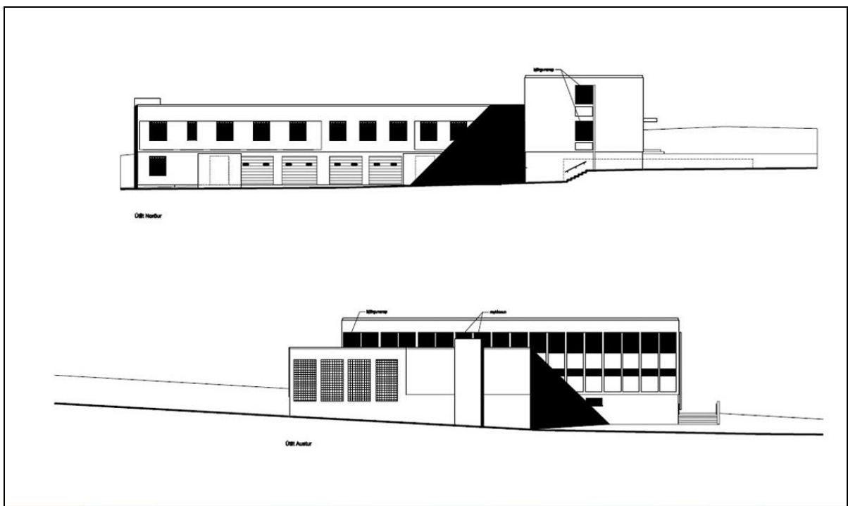
Útlit norður og austur.
