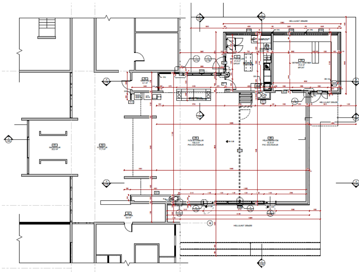
Mynd 1. Grunnmynd viðbyggingarinnar.
